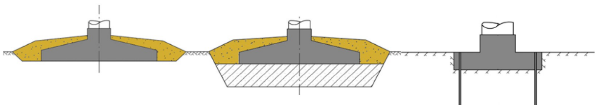
Kuva33: Tuulivoimalat voidaan perustaa useilla eri tavoilla. Periaatekuvat maanvaraisesta teräsbetoniperustuksesta, teräsbetoniperustuksesta massanvaiholla sekä kallioankkuroidusta teräsbetoniperustuksesta.
