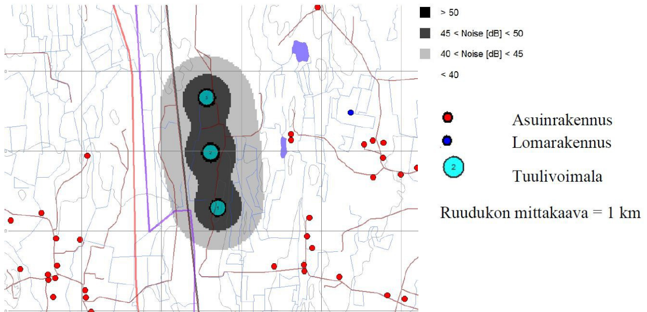
Kuva27: Hankealueelle mahdollisella voimavaihtoehdolla tehty melumallinnus (106 dB)
